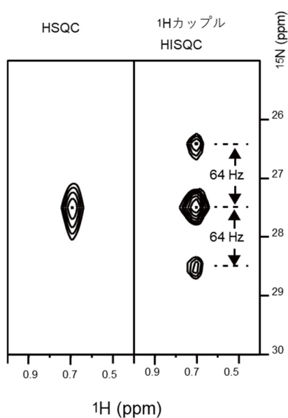
図4 HSQC と HISQC
